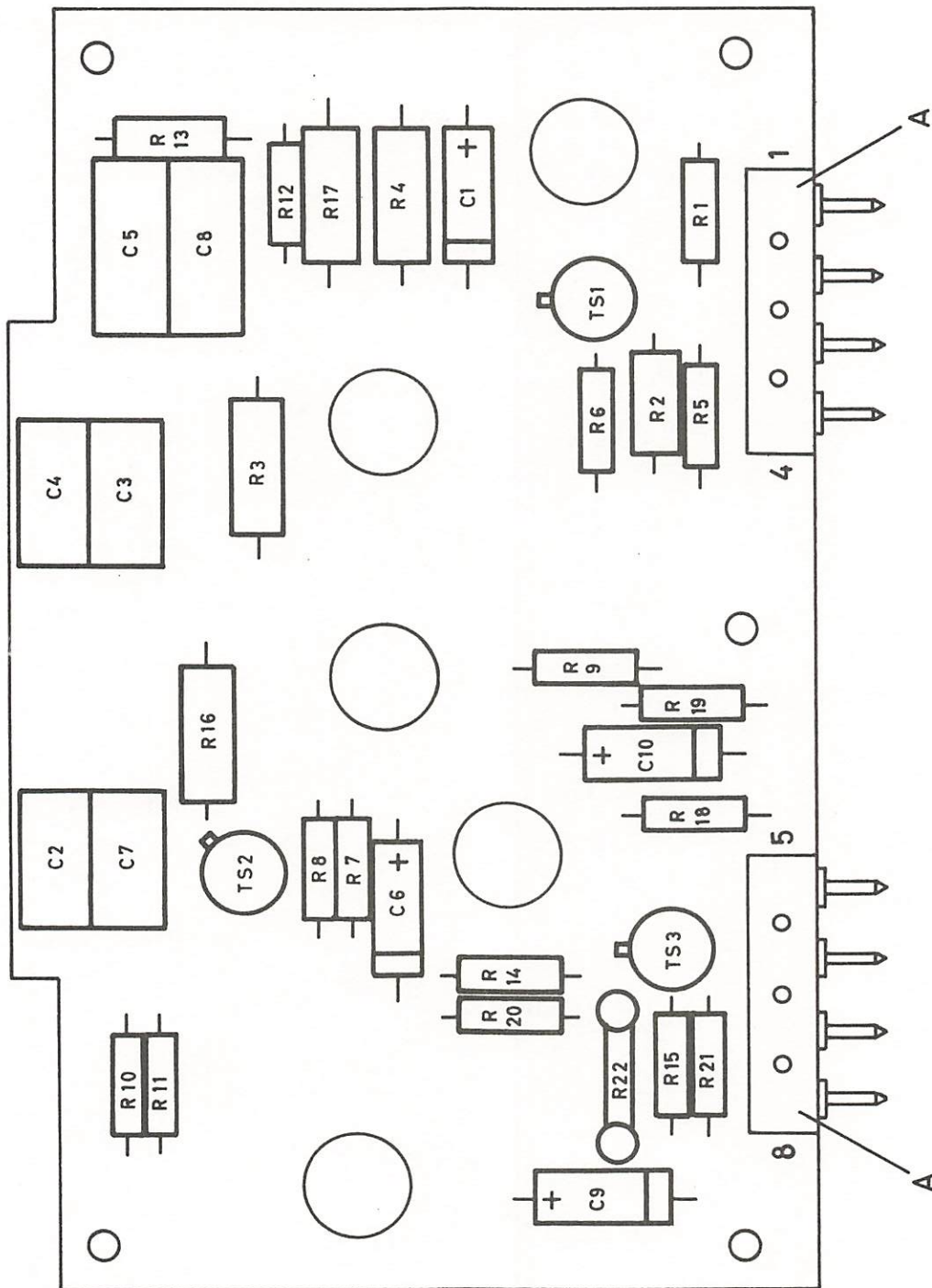
Afb. nr 28 - Toonsquelch, ontvanger; 4B
